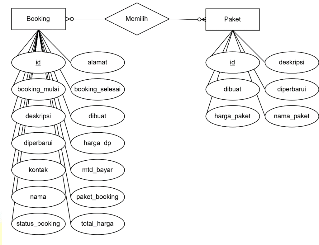
Gambar I - 10. ERD
