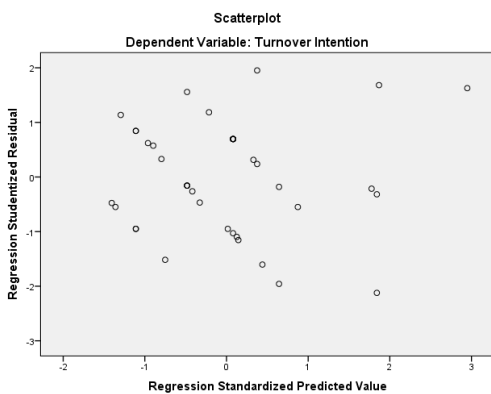
Gambar 2. Uji Heterokedastisitas
