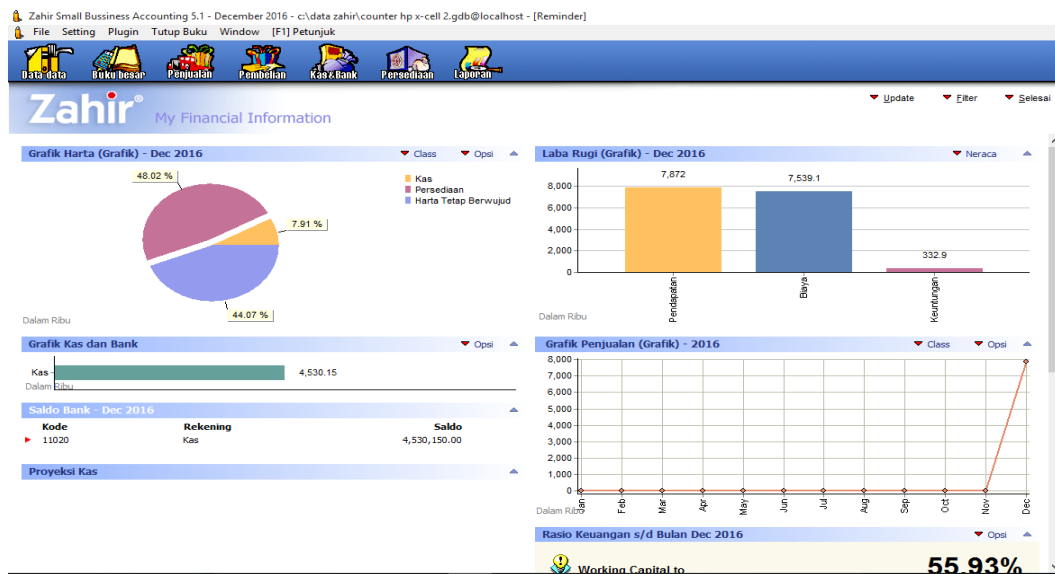
Gambar.10 Analisa Bisnis
