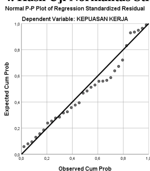
Gambar 4. Hasil Uji Normalitas Struktural I
