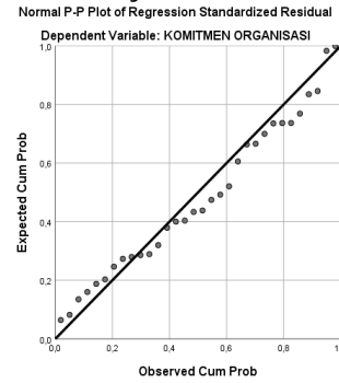
Gambar 5. Hasil Uji Normalitas Struktural II
