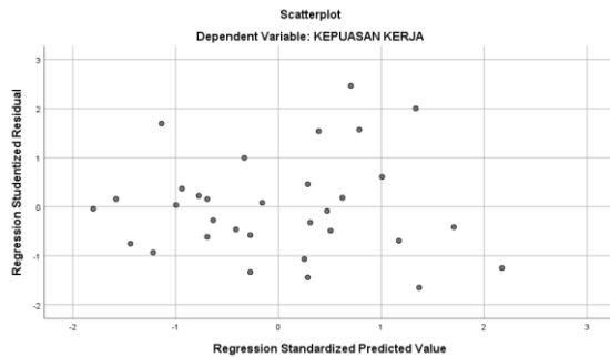
Gambar 3. Hasil Uji Heteroskedastisitas Struktural II
