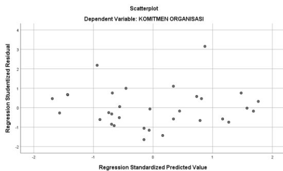
Gambar 3. Hasil Uji Heteroskedastisitas Struktural II
